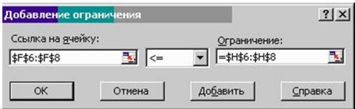
Рис. 4. Добавление ограничения
