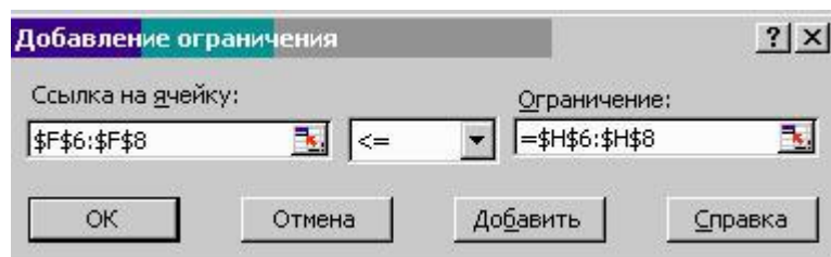
Рис. 4. Добавление ограничения
